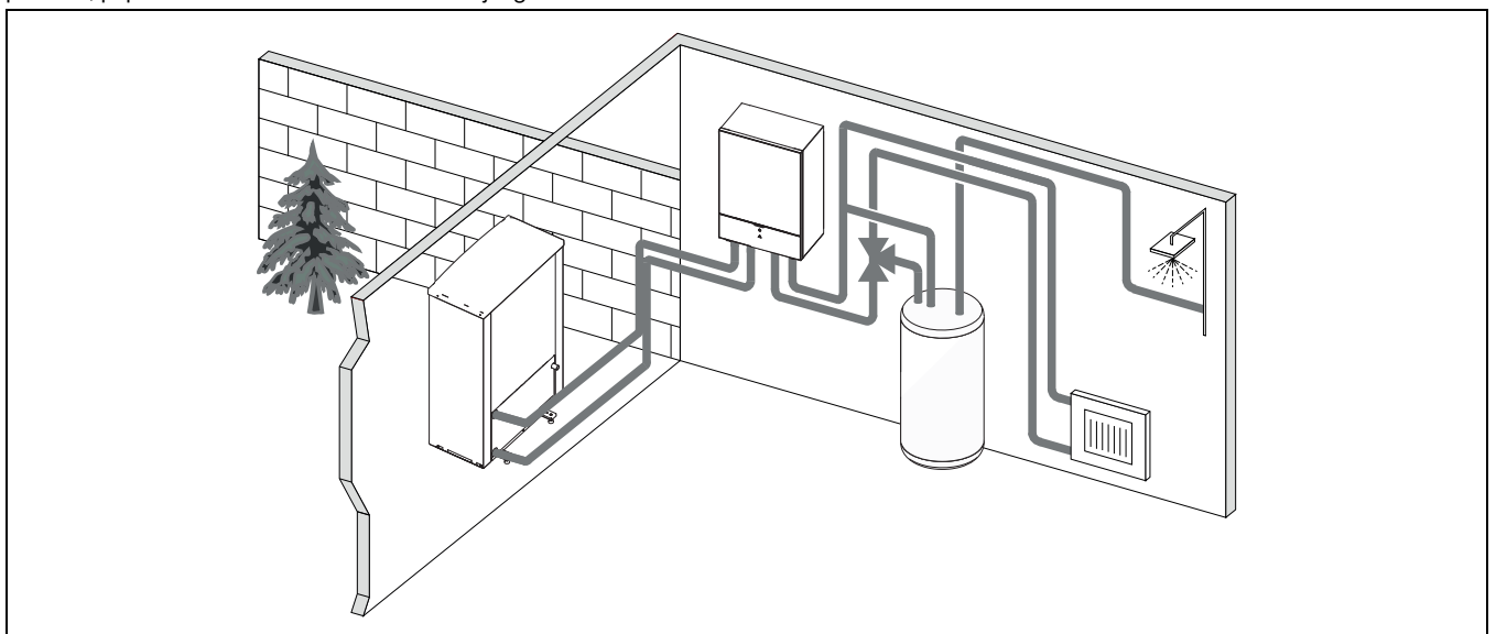
Pav. 3 Šilumos siurblys Compress 7000i AW, vidinis blokas AWE su elektriniu kaitintuvu ir išorine karšto vandens talpykla
