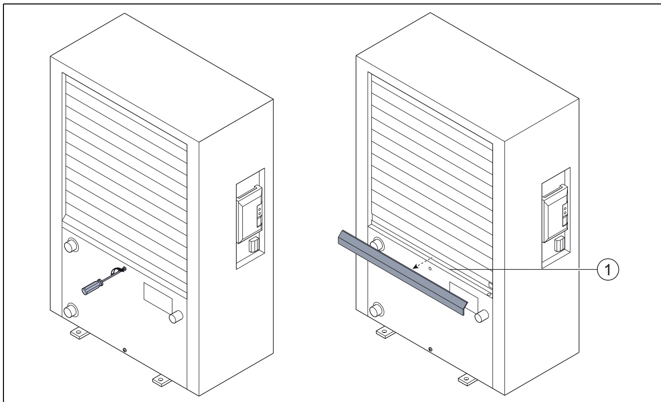
Pav. 9 Šilumos siurblio kondensato vonelė
