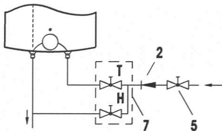
Otevřený (průtokový) systém
