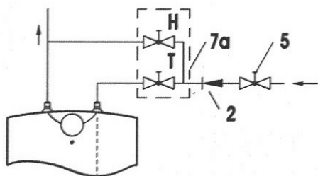
Provedení pod odběrné místo
