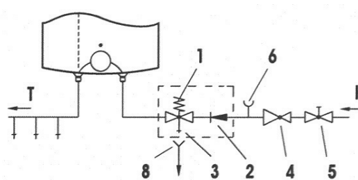
Uzavřený (tlakový) systém
