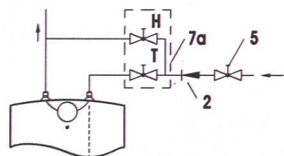
Исполнение под точкой отбора
