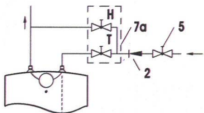
Prevedenie pod odberné miesto
